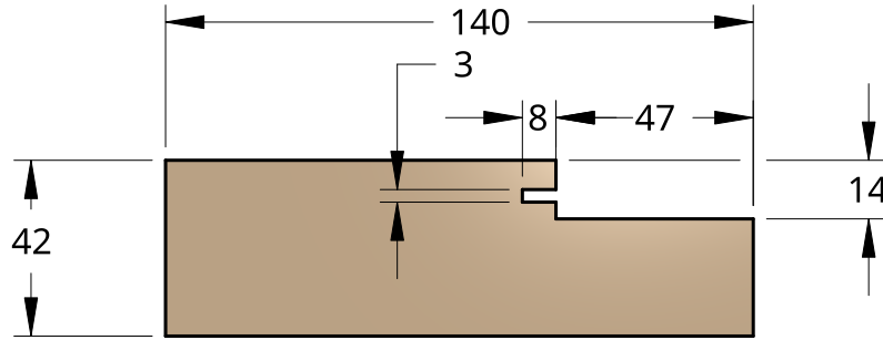
JAMB
